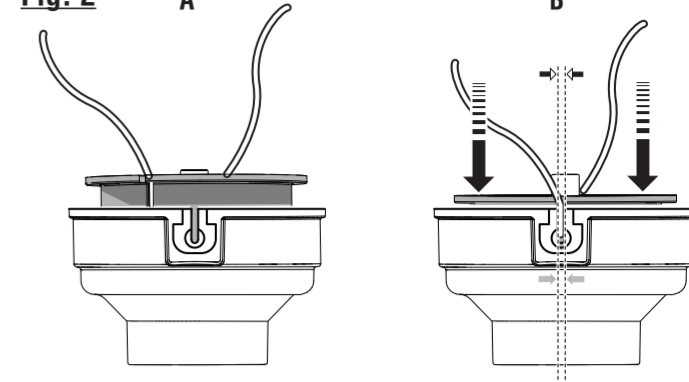
A - Insert line into string head (insérer dans l'extrémité de la chaîne, insérer en el cabezal del hilo) B - Push down and twist to align (pousser vers le bas et tordre pour aligner, empujar hacia abajo y gire para alinear)
